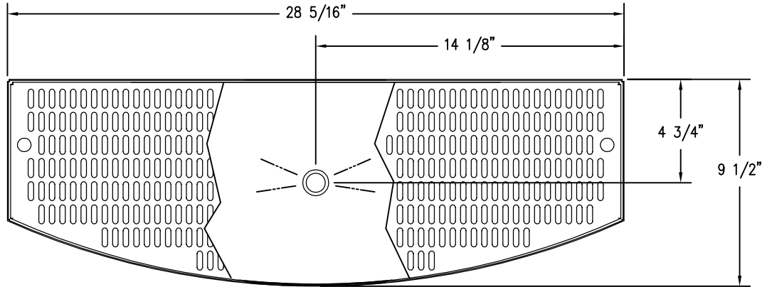
DRAINER: 71-0028-99
