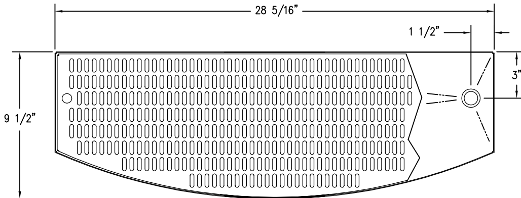
DRAINER: 71-0028-99-R
