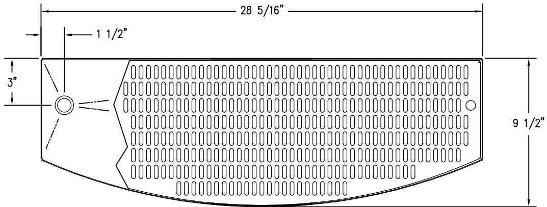
DRAINER: 71-0028-99-L
